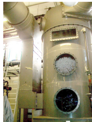
Abluftleistung 15.000 m 3 /h
